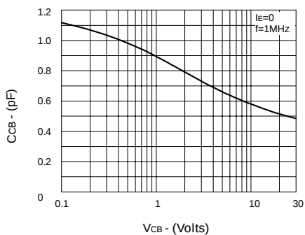
C_{CB} v V_{CB}
